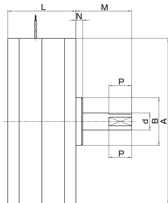
シャフト断面
