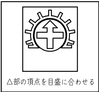
内蔵半固定VR拡大図
