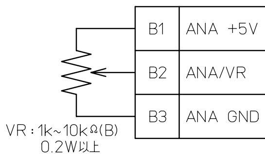
サブ設定入力：外付けVR接続
