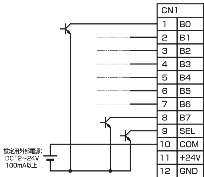
デジタル設定入力接続 外部電源を使用する場合
