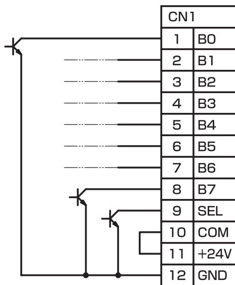
デジタル設定入力接続 デジタル設定入力専用電源を使用する場合
